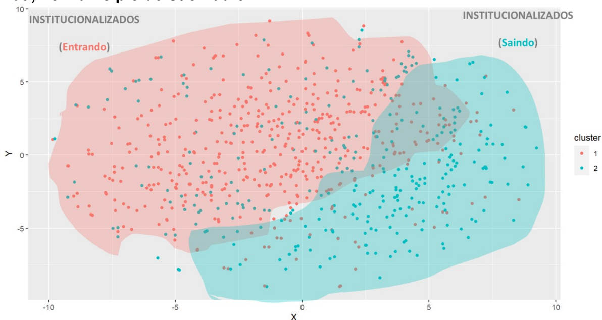
Figura 19 - Denominações dos Cluster a Partir das Nuvem de Pontos do Clusters 1, em 2 Subclusters dos Perfis Socioeconômicos da População em Situação de Rua, no Município de São Paulo.
