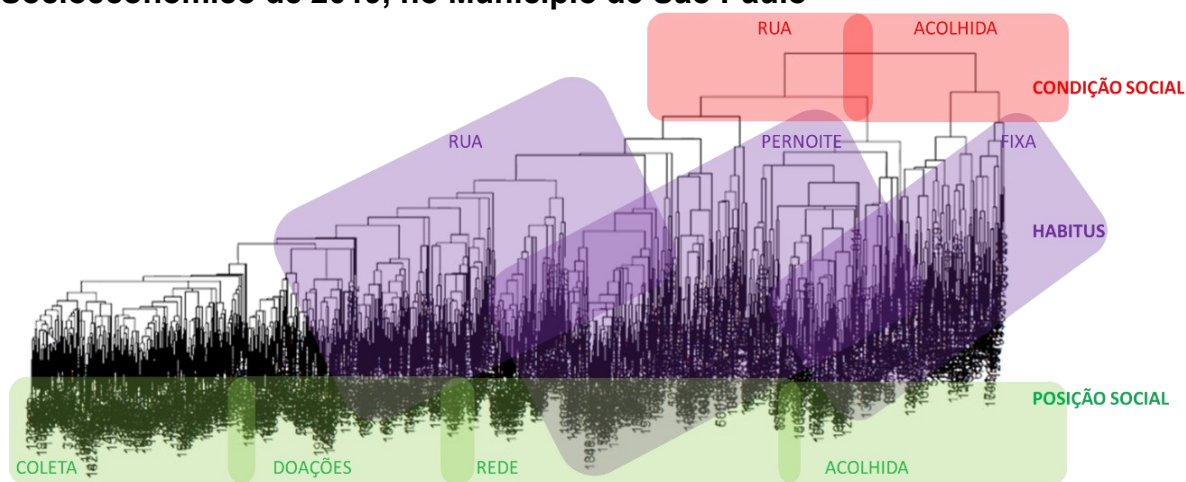
Figura 16 - Ilustração da Condição e Posição dos Sujeitos em Situação de rua A Partir de Dendrograma Hierárquico, Pesquisa Amostral de Perfil Socioeconômico de 2019, no Município de São Paulo
