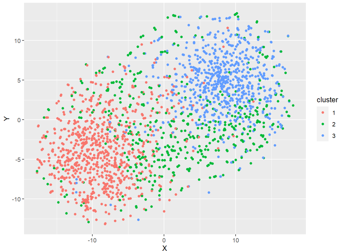
Gráfico 7 - Nuvem de Pontos de 3 Clusters
