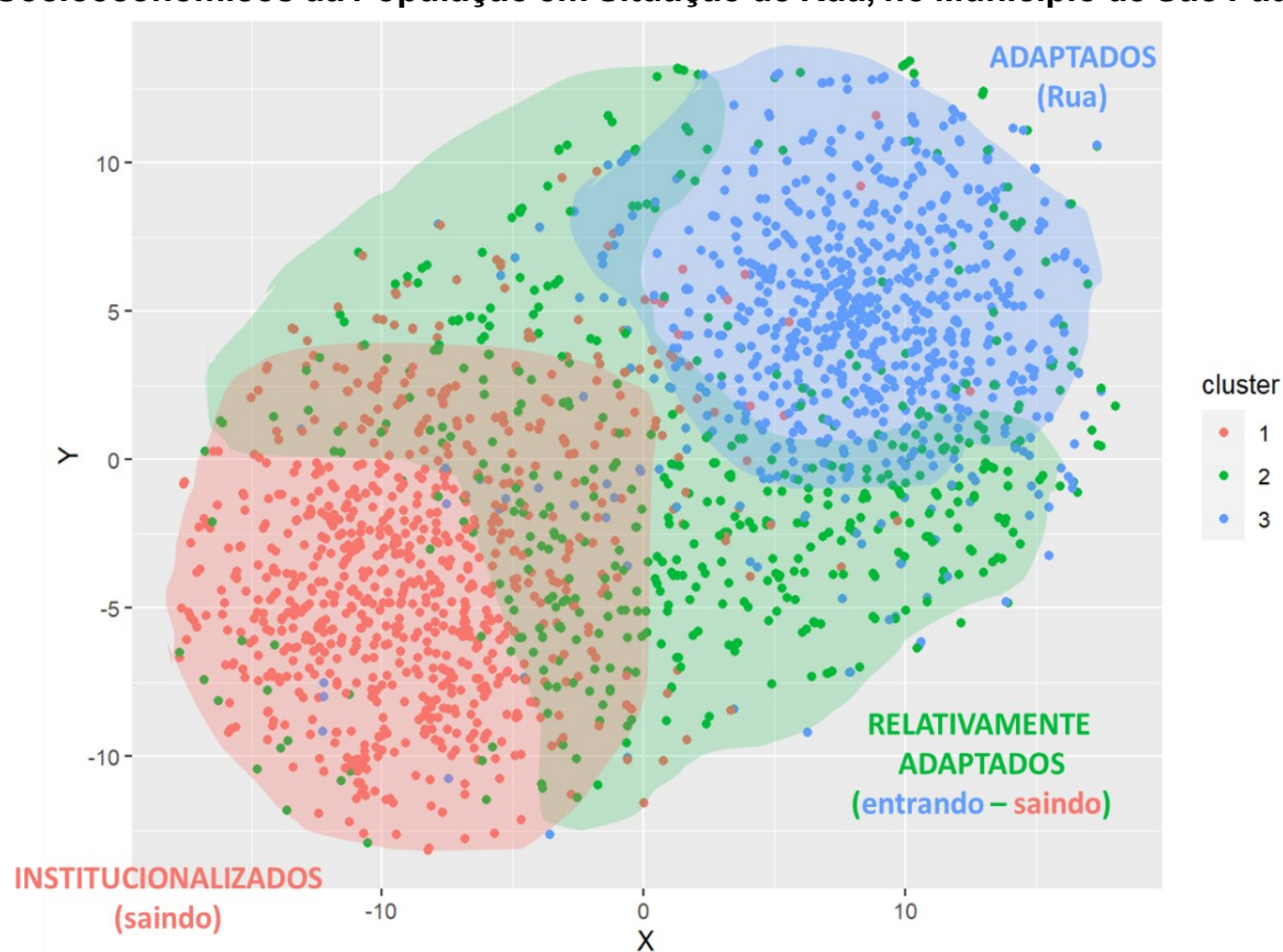
Figura 18 - Denominações dos Cluster a Partir das Nuvem de Pontos dos Perfis Socioeconômicos da População em Situação de Rua, no Município de São Paulo
