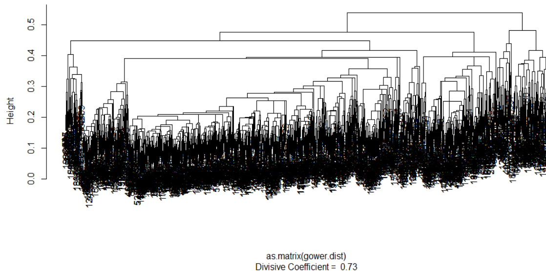
Figura 17 - Matriz de componentes principais com clusters hierárquicos, do Perfil Socioeconômica da População em Situação de Rua de São Paulo, em 2019
