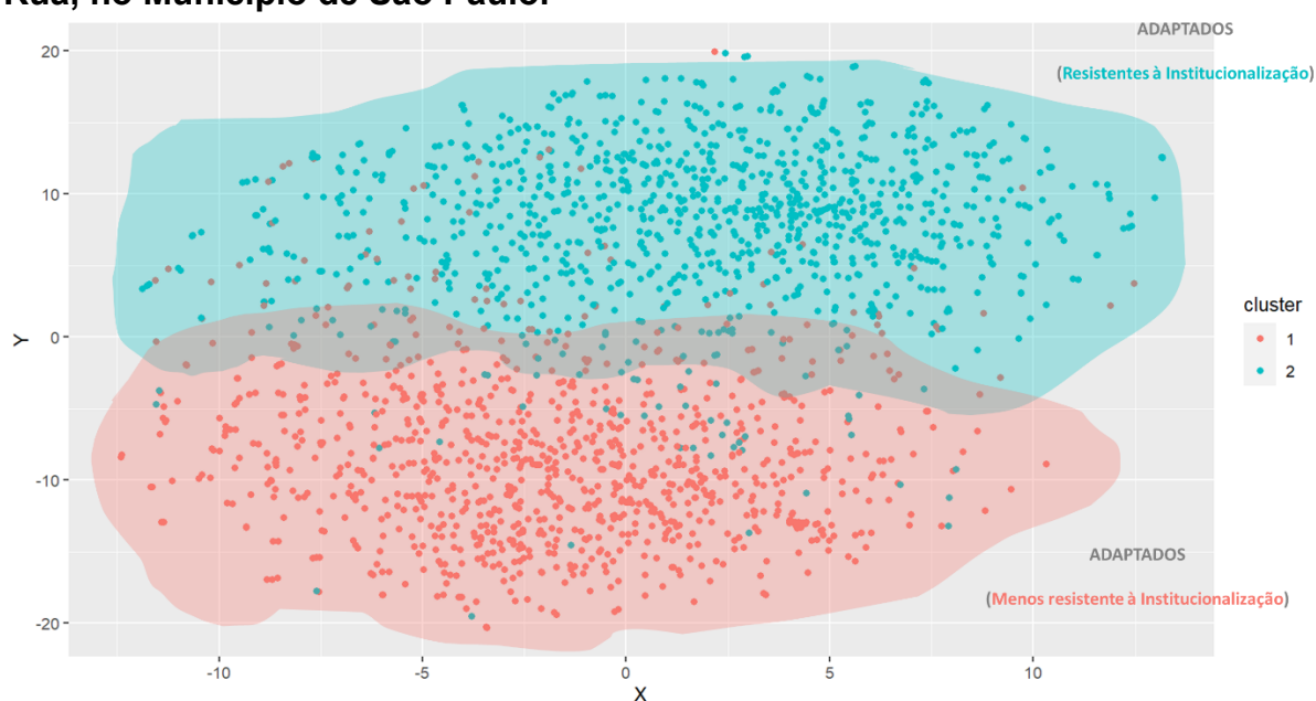
Figura 20 - Denominações dos Cluster a Partir das Nuvem de Pontos do Clusters 3, em 2 Subclusters dos Perfis Socioeconômicos da População em Situação de Rua, no Município de São Paulo.
